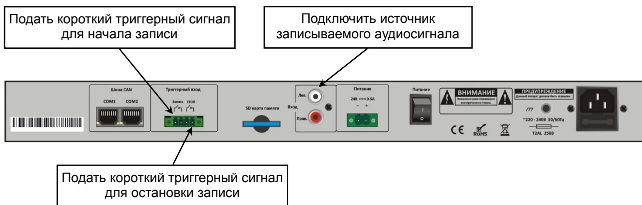
Рис. 4.1. Порядок управления блоком записи сообщений LPA-EVA-RC
